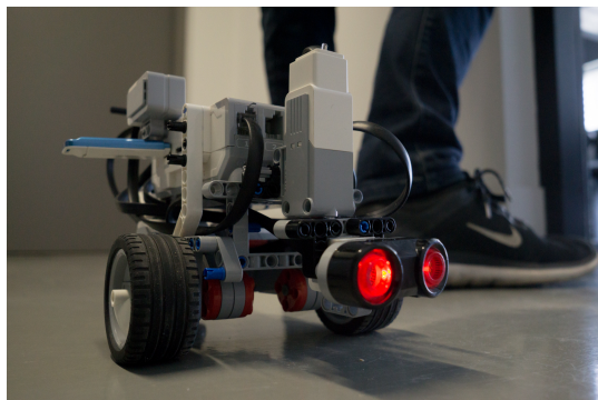
Projekt v rámci jednoho z předmětů – autonomní robot LEGO Mindstorms schopný mapovat projeté území
